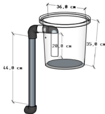
Gambar 1. Desain CSD tampak samping
